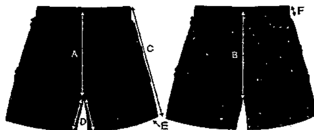
Medidas do short sem a saia
