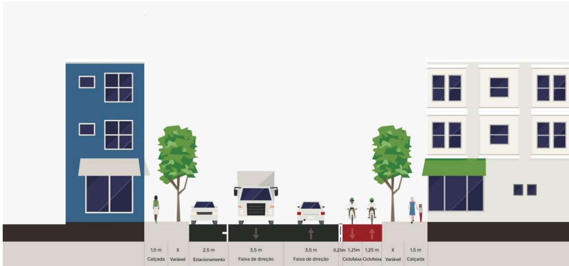
DESENHO 04 – Dimensionamento das Vias Arteriais
